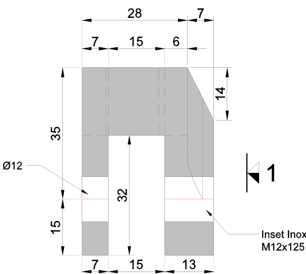
Coupe A-A Ech: 1/1
